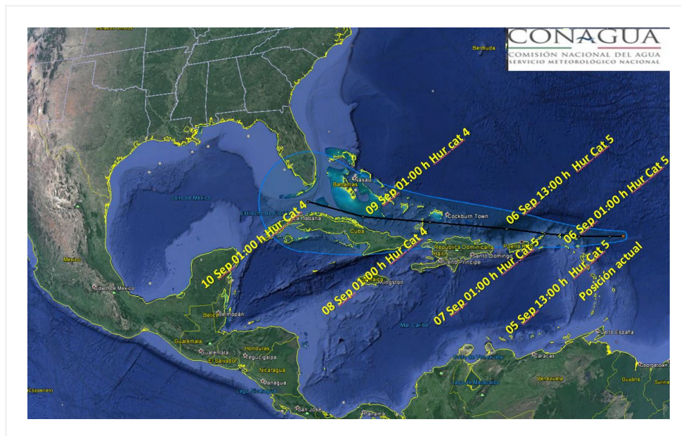
Traectoria pronóstico del Huracán IRMA Categoría 5.
